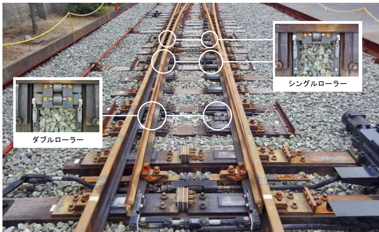
オーストロロール設置例 (60K12番弾性ポイント)
